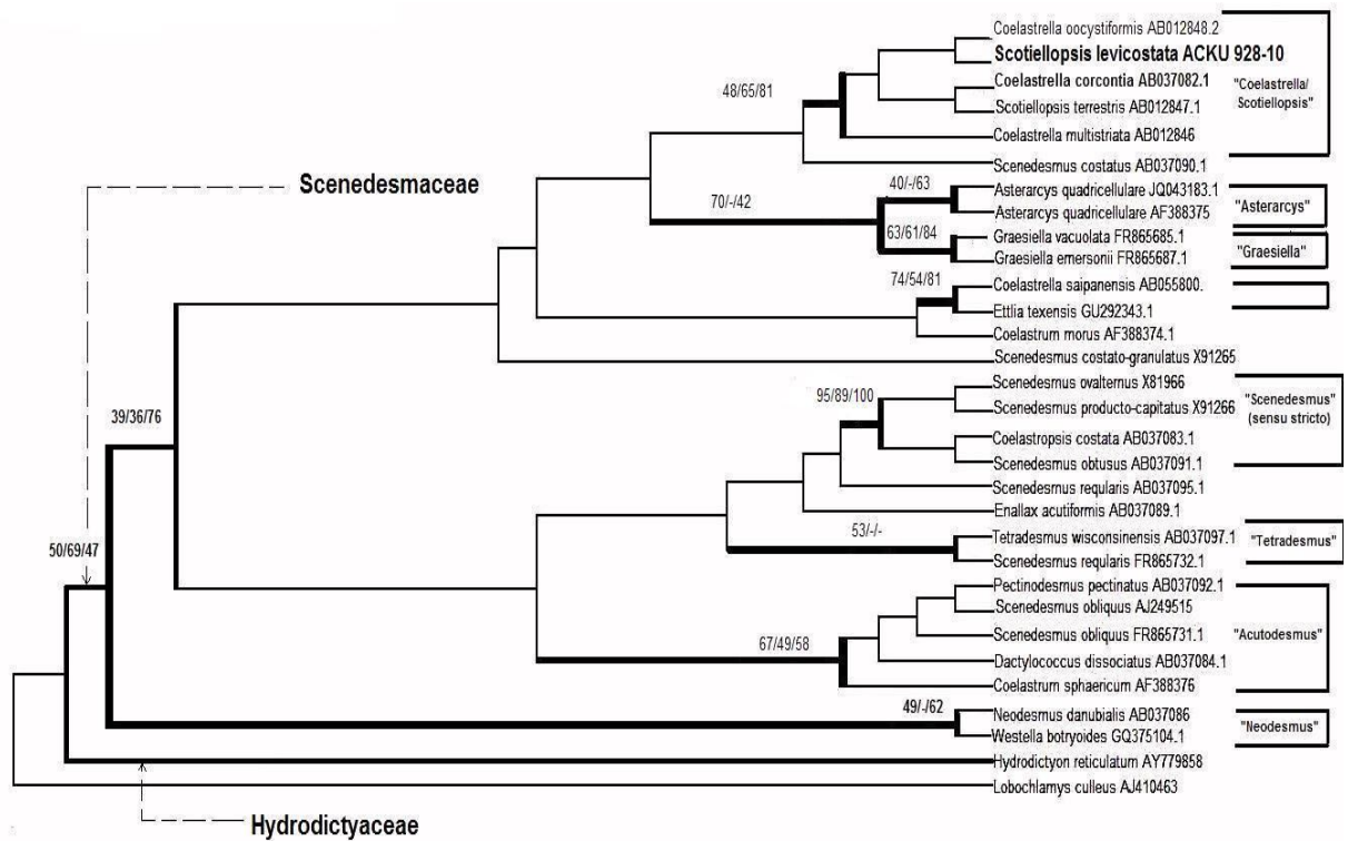
Рис. 3. Місце Scotiellopsis levicostata (штам ACKU 928-10) в системі Scenedesmaceae за результатами аналізу послідовностей 18S рДНК (філогенетичне дерево, що побудовано за ML- методом; на гілках - значення бутстрепа для ML/MP/NJ дерев. Гілки, які хоча б за одним методом мають підтримку вищу за 50%, виділені товстими лініями).
